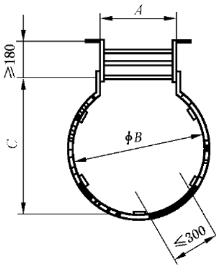
a) 圆形护笼中间笼箍
