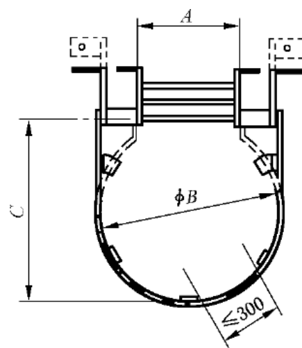
b) 圆形护笼顶部笼箍
